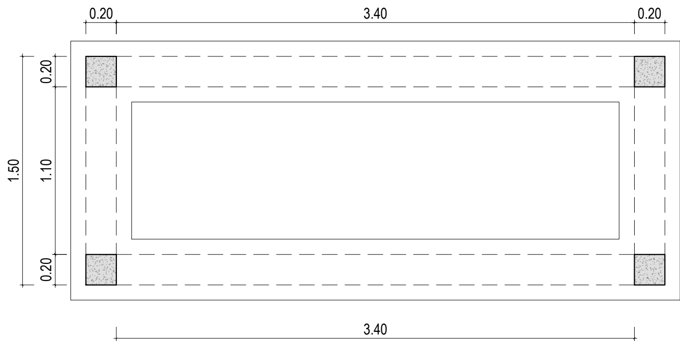
Detalhe – pilaretes escala 1/25
