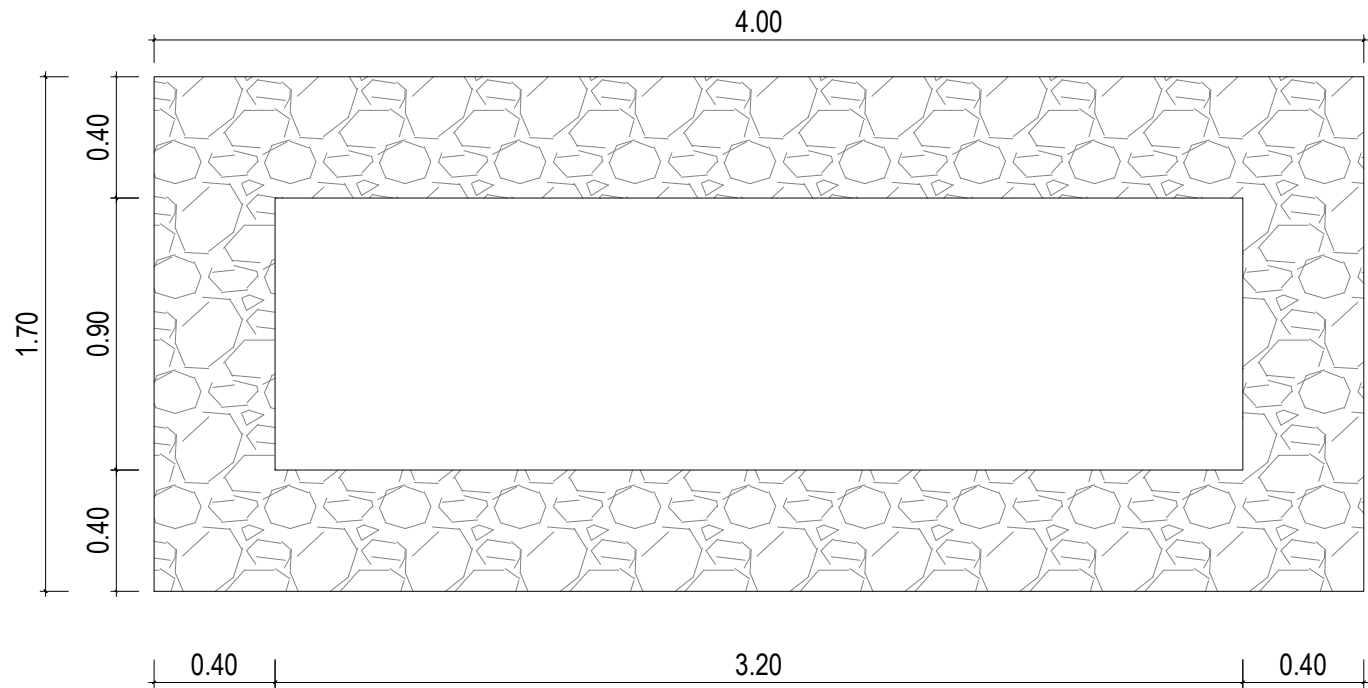
Detalhe – emb. em pedra argamassada escala 1/25
