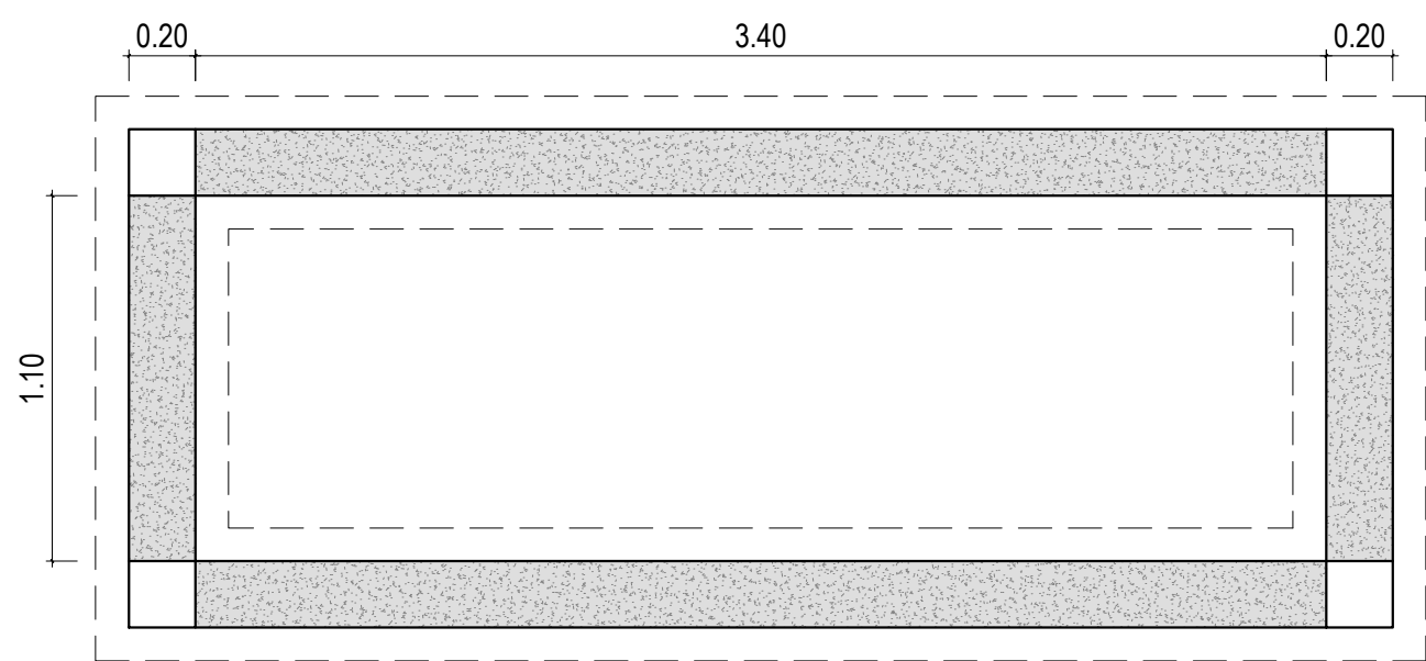
Detalhe – Cintas escala 1/25
